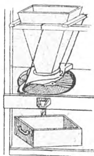
18. Coșul morii. (Jos, lădița în care curge făina).
